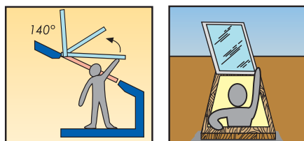
Apertura a ribalta fino a 140°
