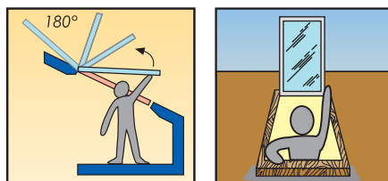
Apertura a ribalta fino a 180°
